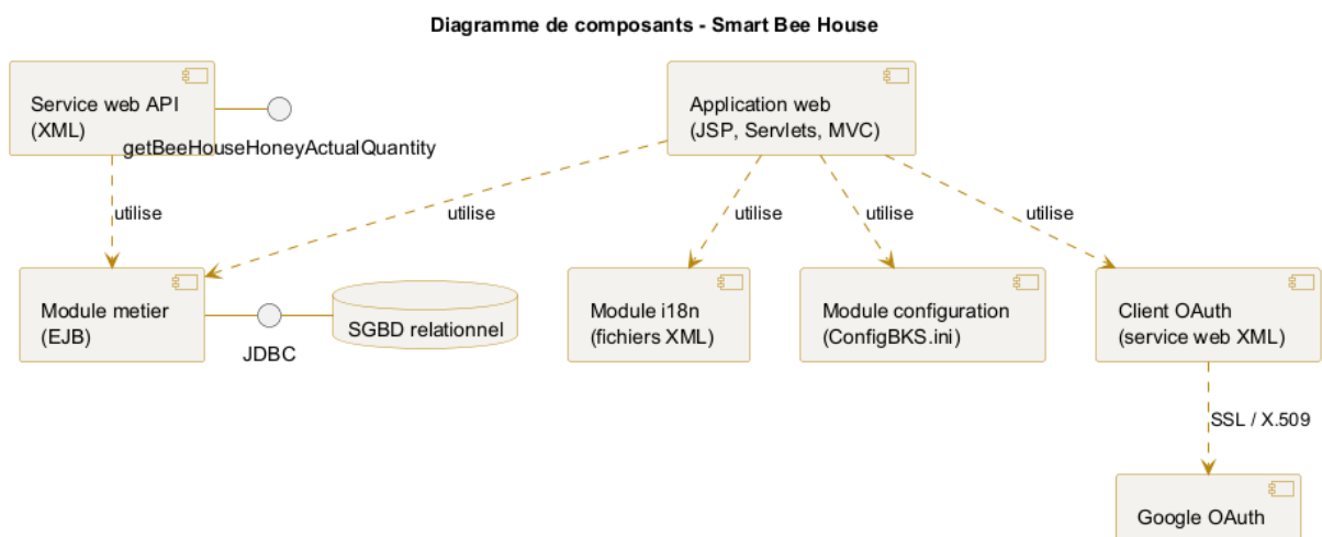
Figure 7.9. Diagramme de composants du système Smart Bee House.
