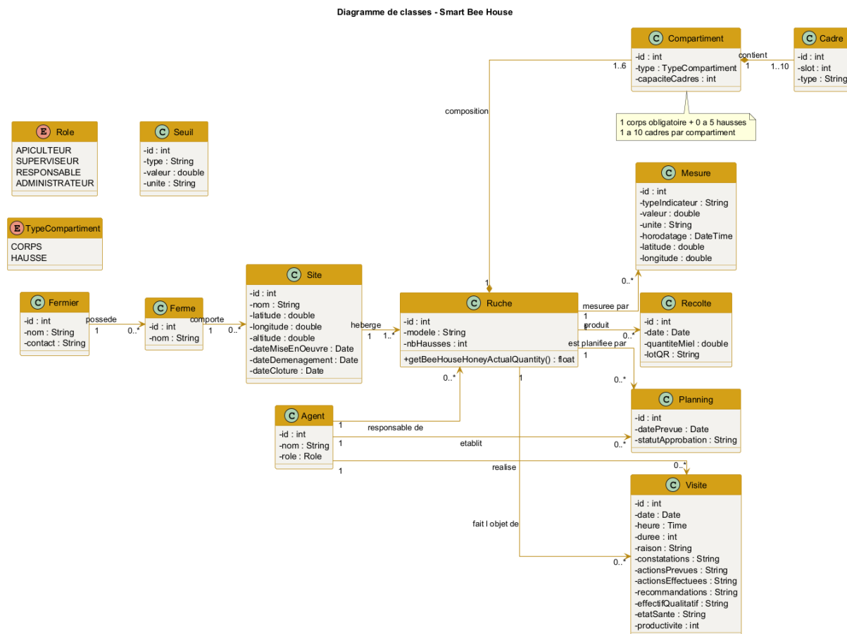
Figure 7.1. Diagramme de classes du système Smart Bee House (alignement horizontal).
