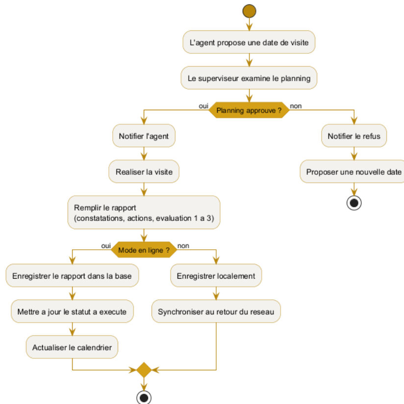
Figure 7.6. Diagramme d'activité du processus de visite.
