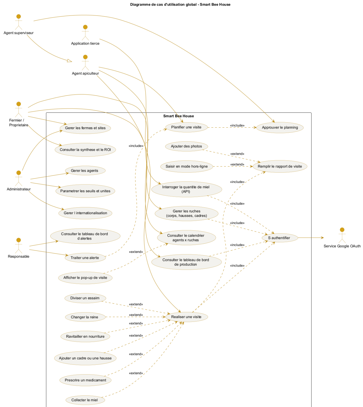
Figure 6.1. Diagramme de cas d'utilisation global avec acteurs et dépendances (include et extend).
