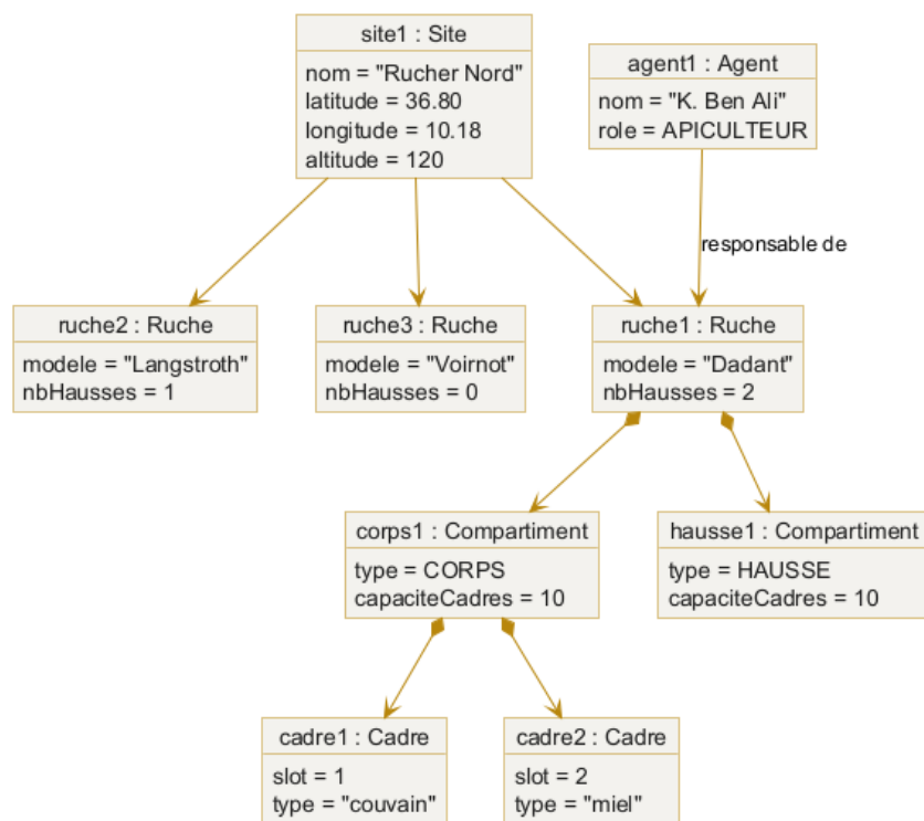
Figure 7.5. Diagramme d'objets, instantané d'un site apicole.
